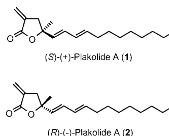
Figure 1. ( S )-(+)-Plakolide A and ( R )-(-)-Plakolide A.
